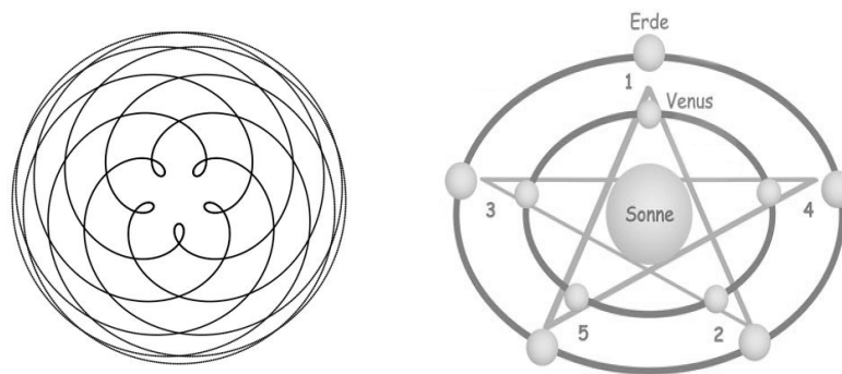
DIE VENUSUMLAUFBAHN
